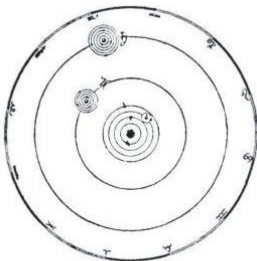
Fig. V.- Sistema de Copérnico.
